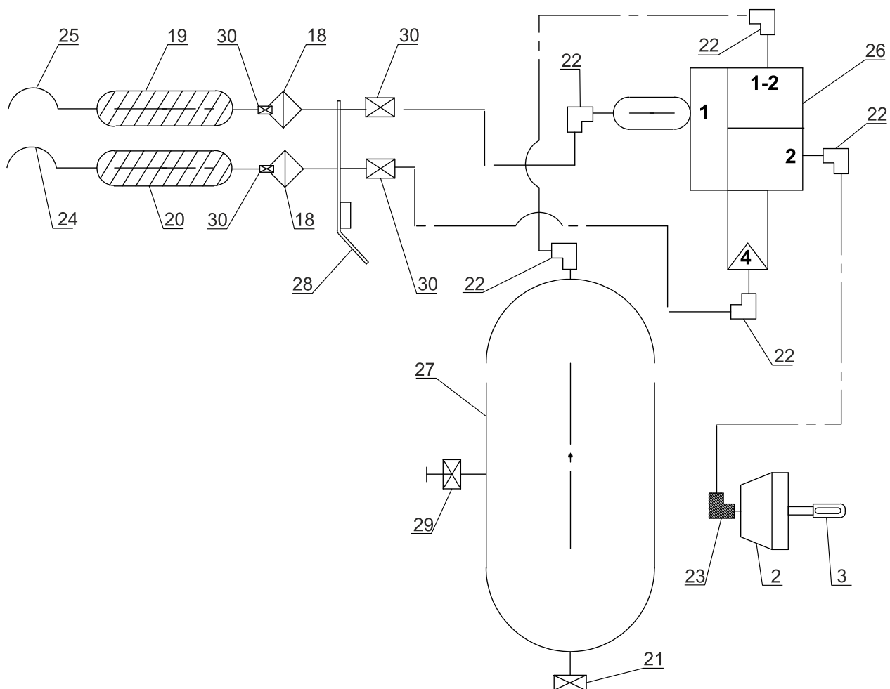
Schemat instalacji pneumatycznej układu hamowania
