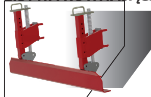
przednia LISTWA RÓWNAJĄCA
